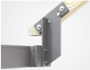
Dachsparrenmontage
